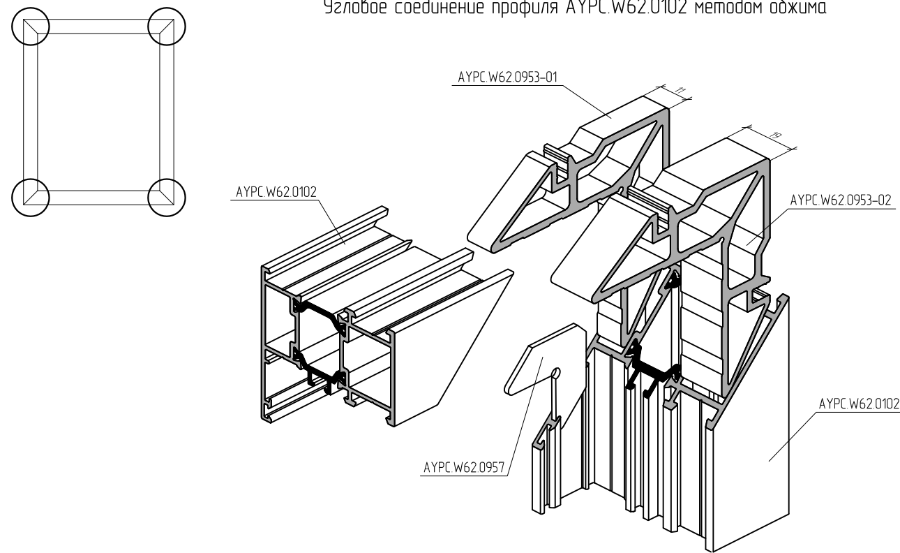
Узловое соединение профиля АУРС.W62.0102 методом обжима
