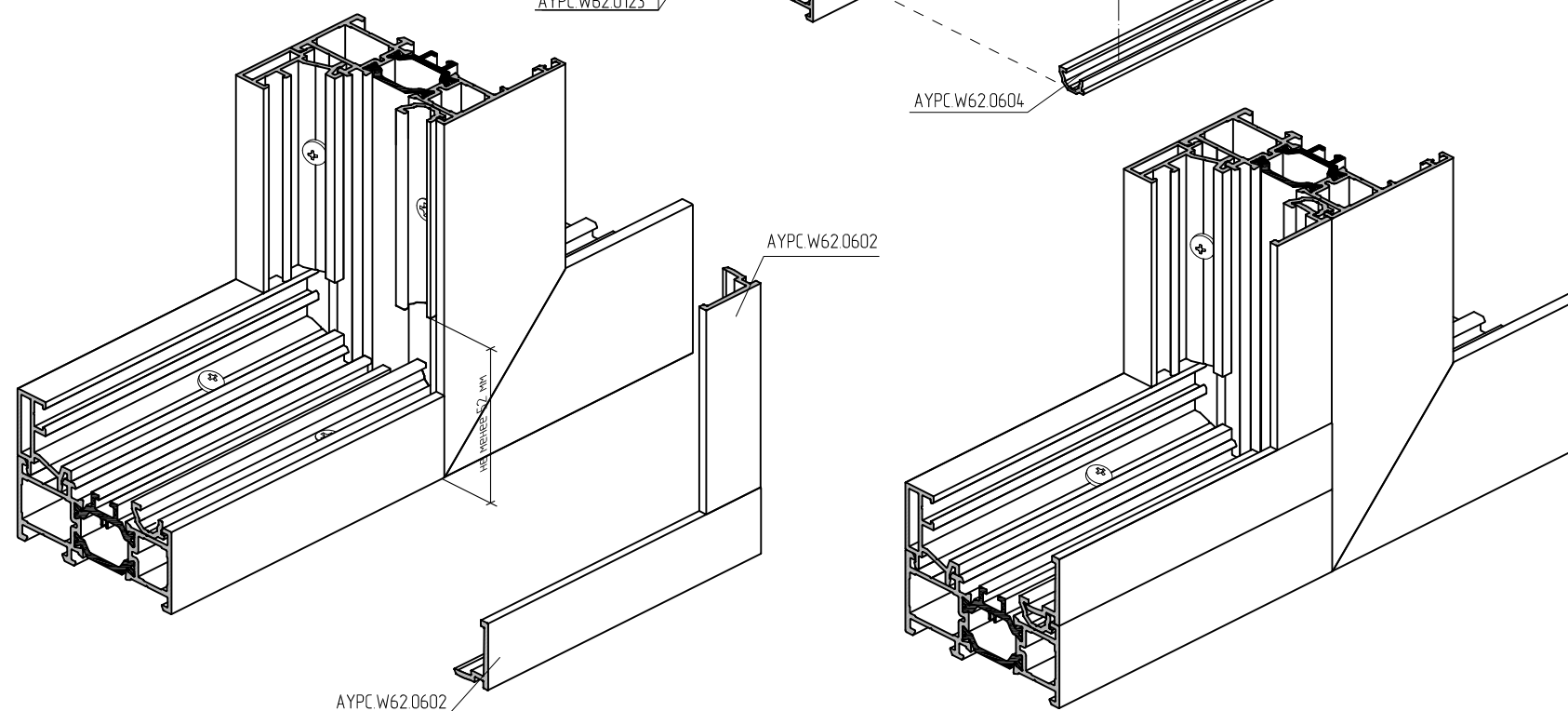
Схема установки профиля АУРС.W62.0604 (только для вертикальных профилей)
