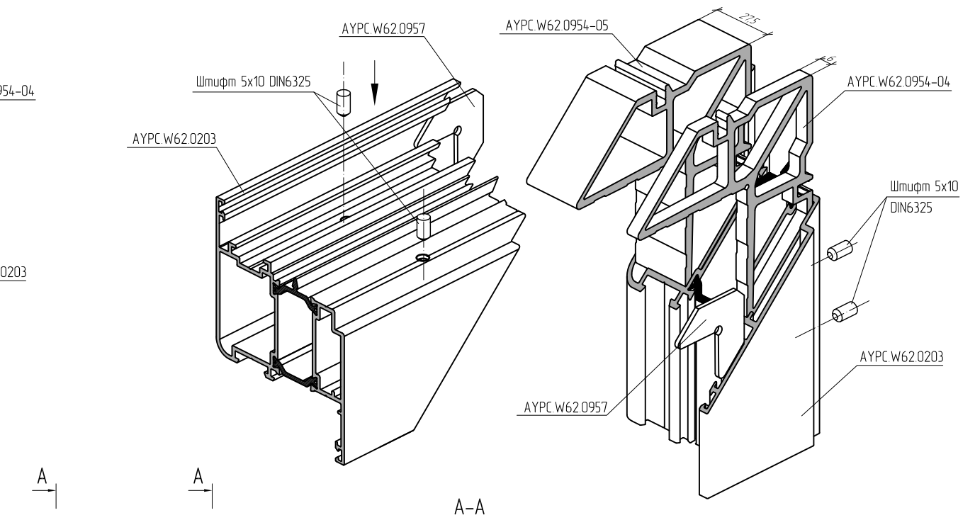
Узловое соединение профилей АУРС.W62.0203 с использованием штифтов 5x10
