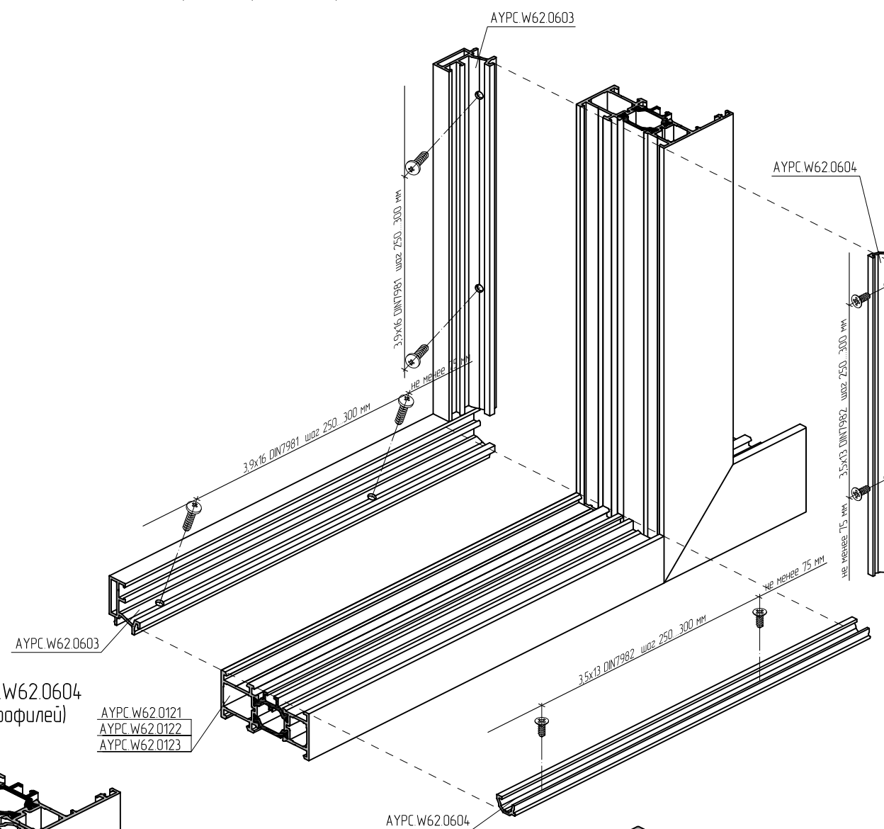
Сборка и обработка простеночной части ленточного остекления
