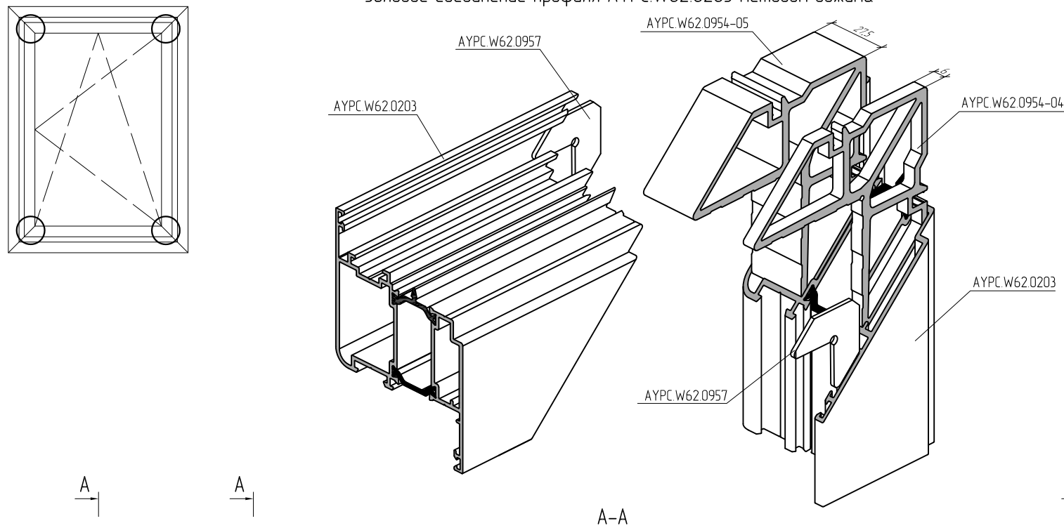
Узловое соединение профиля АУРС.W62.0203 методом обжима
