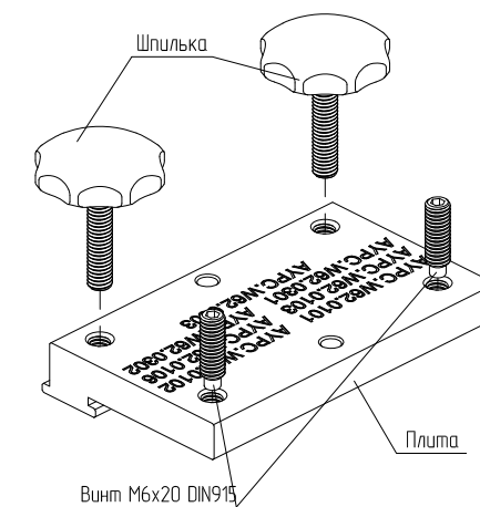
Кондуктор АУРС.W62.1940
