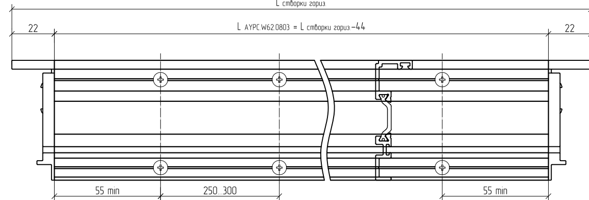
Схема установки профиля AYPC W62.0803.
