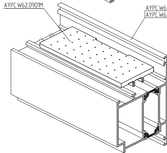
Подкладка опорная AYPC.W62.0901M
