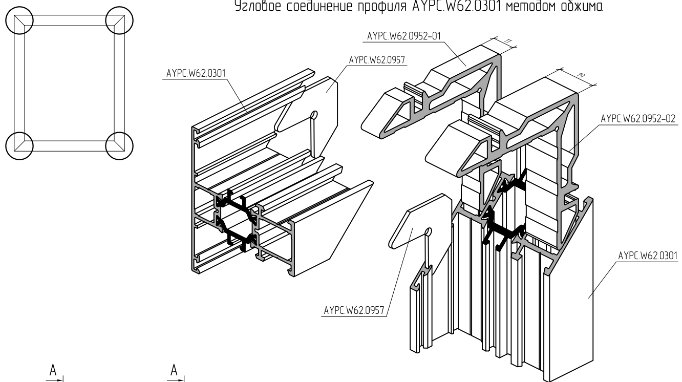
Угловое соединение профиля АУРС.W62.0301 методом обжима
