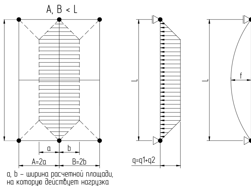
Рис. 4. Схема нагрузок
