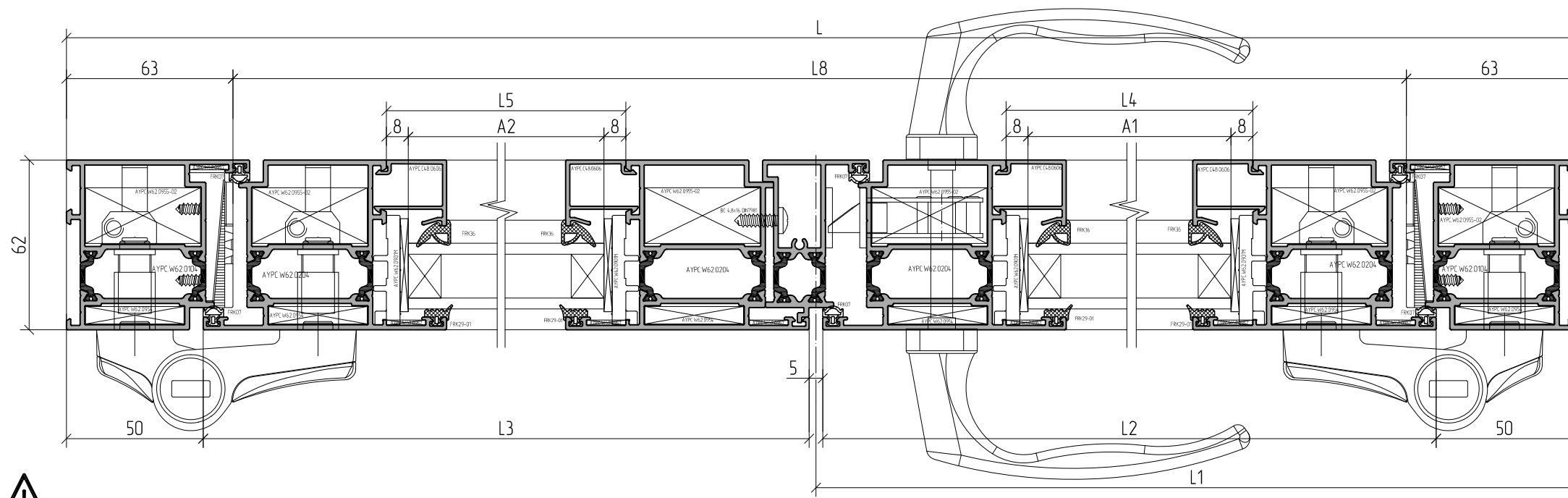
A-A
