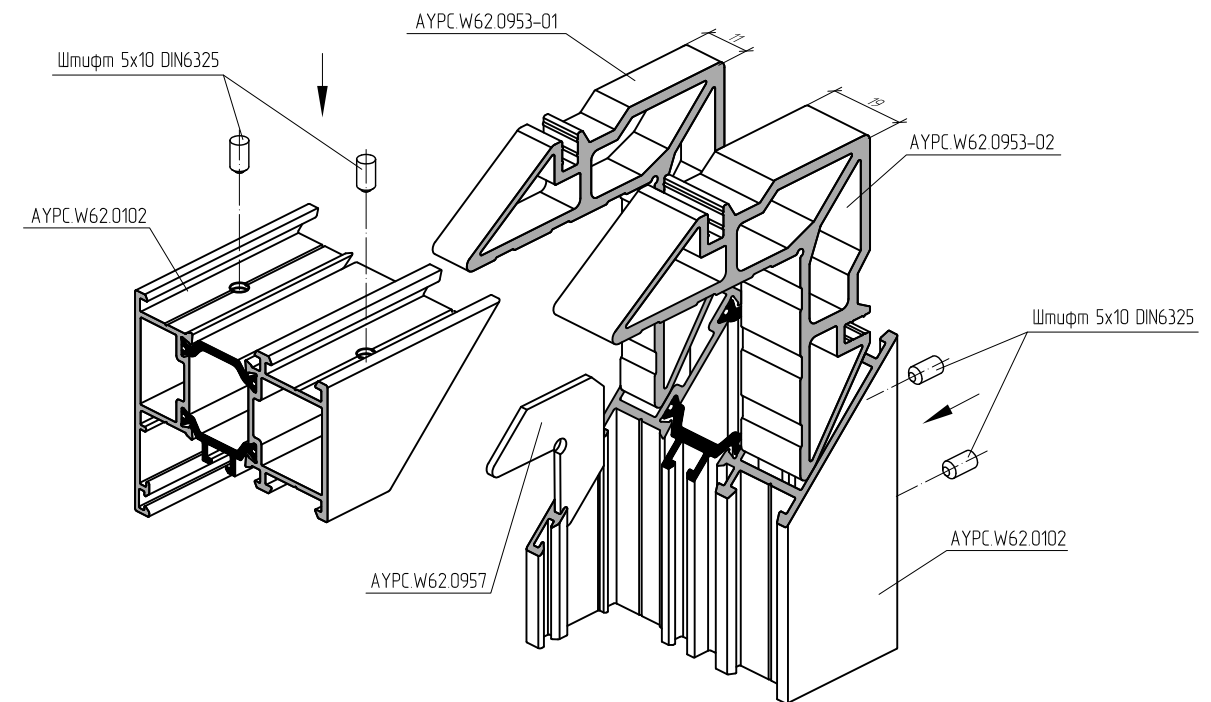
Узловое соединение профиля АУРС.W62.0102 с использованием штифтов 5x10
