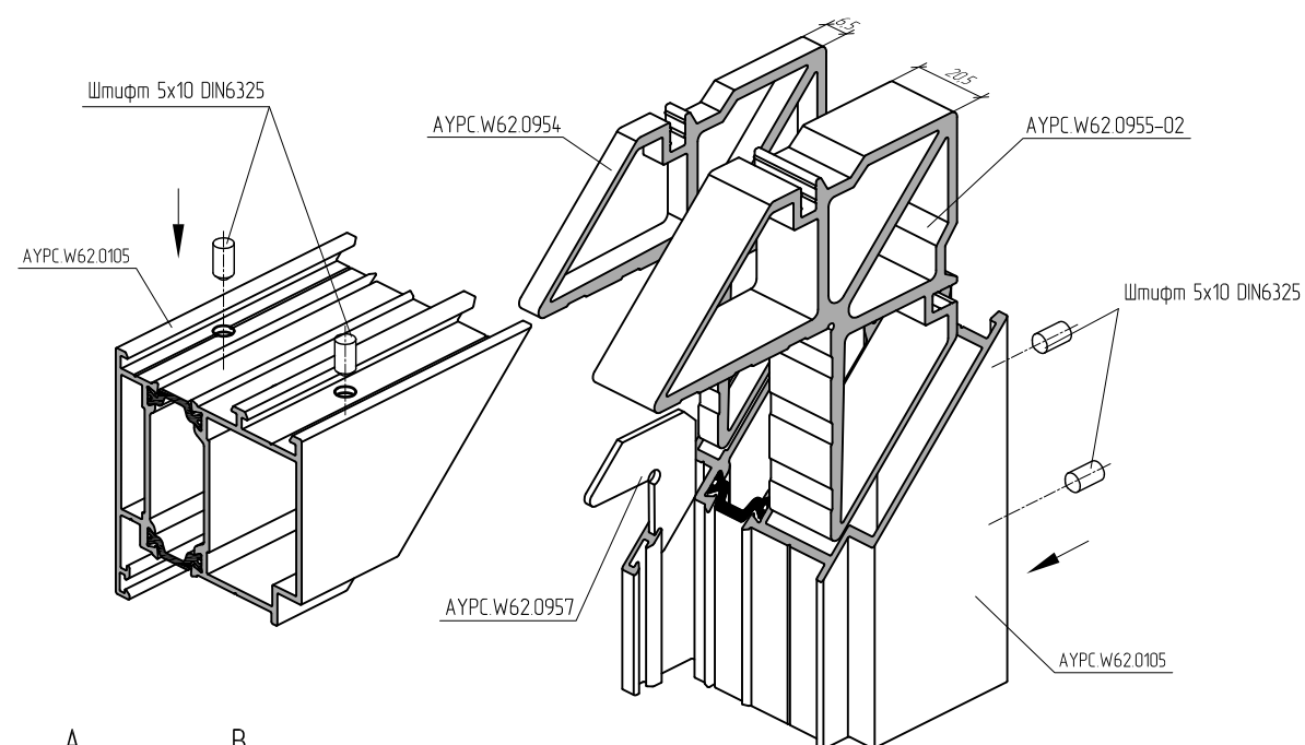
Угловое соединение профилей АУРС.W62.0105 с использованием штифтов 5x10. Вариант 2
