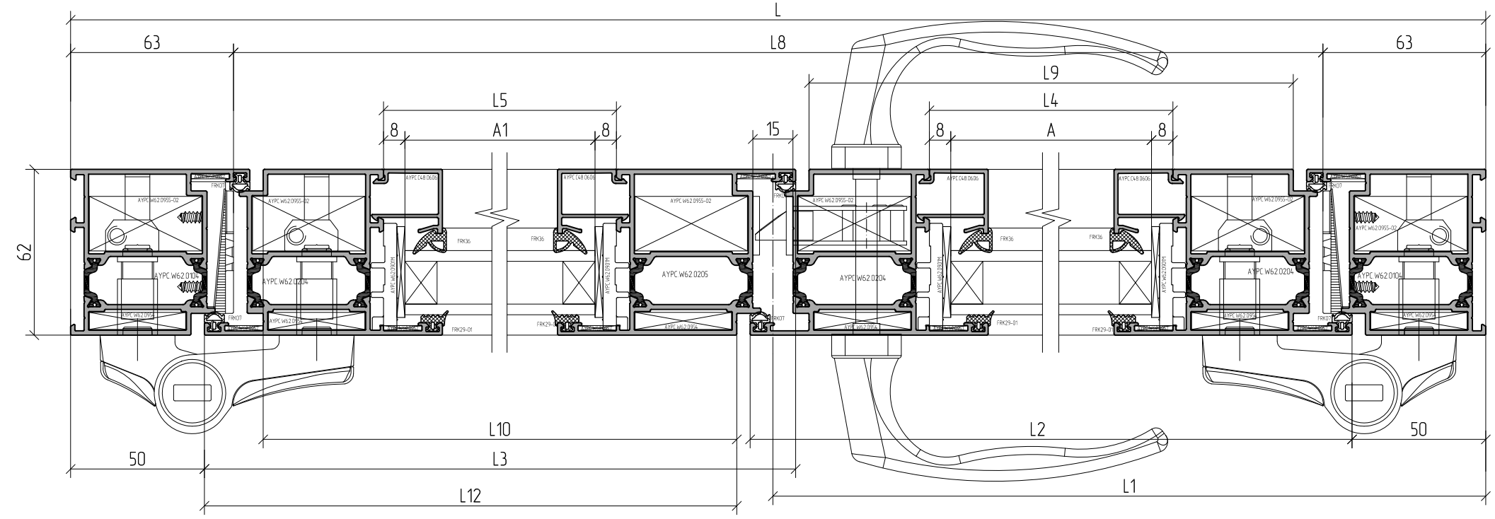
A-A
